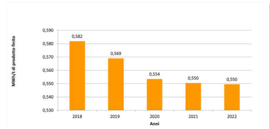
Grafico 5 - Consumi specifici di energia elettrica
