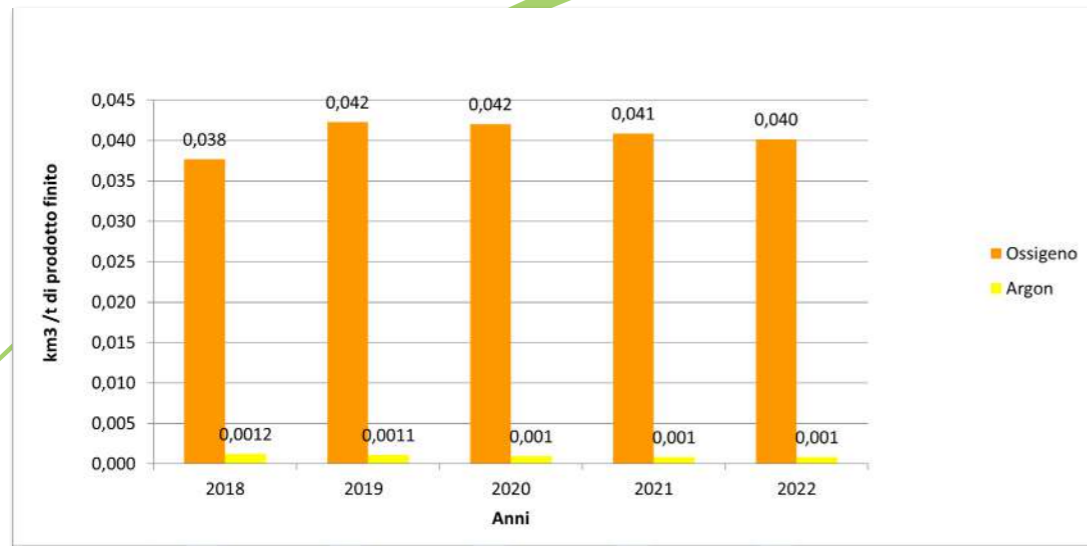
Grafico 4 - Consumi specifici di ossigeno e gas
