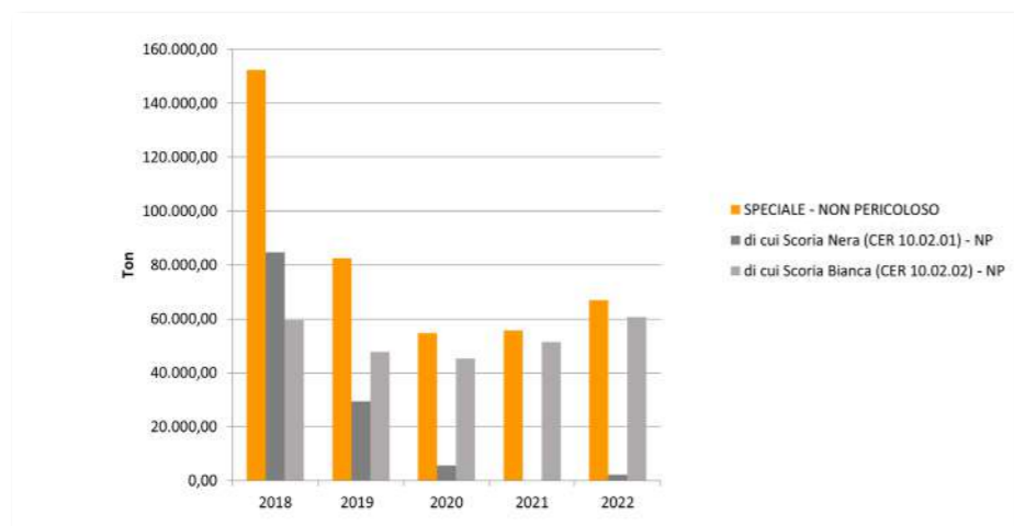
Grafico 16 - Rifiuti non pericolosi
