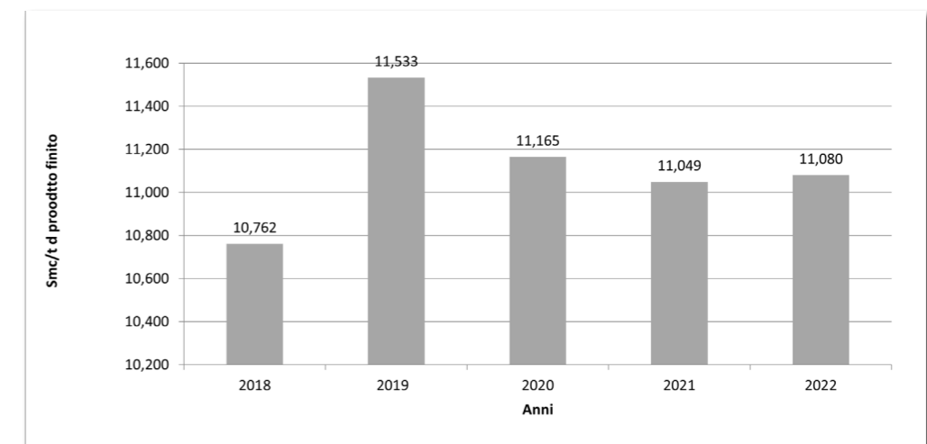
Grafico 6 - Consumi specifici di gas naturale
