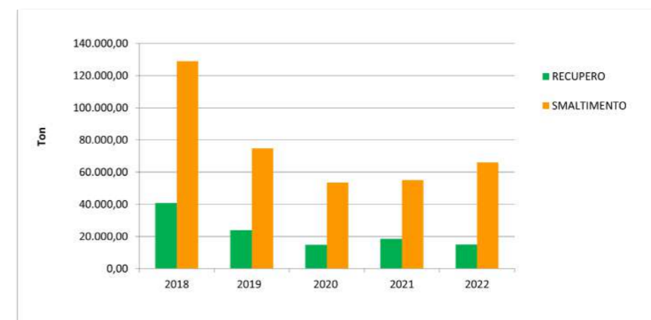
Grafico 17 - Recupero vs smaltimento
