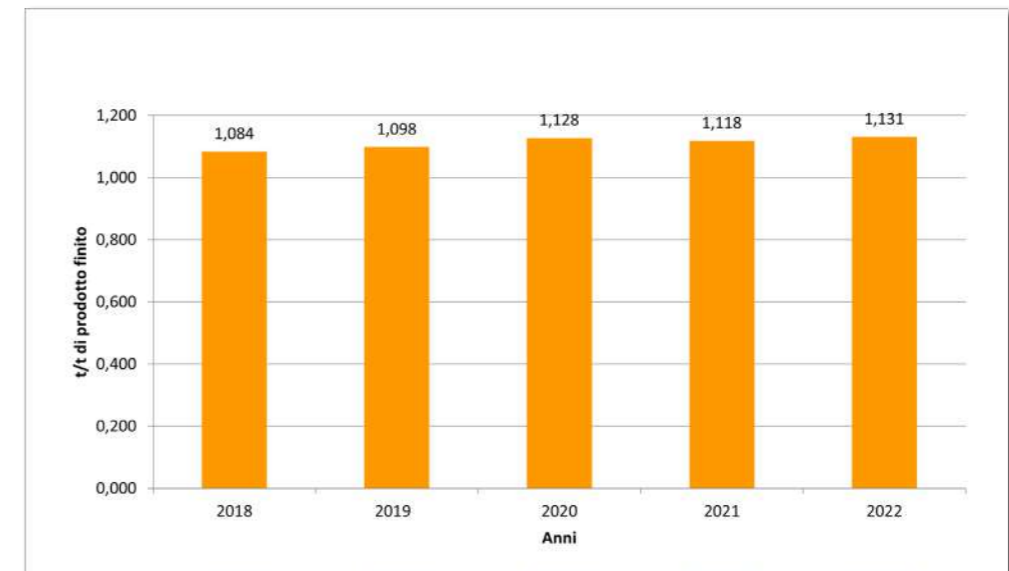
Grafico 2 - Consumi specifici di rottame di ferro
